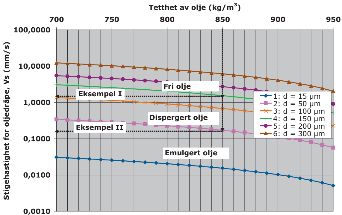
Figur 3.1 Stigehastighet i stillestående vann for oljedråper med ulike diameterer og tetthet (Beregnet ved hjelp av Stokes lov, Kinematisk viskositet for vann: 1,2 \cdot 10^{-6} \text{ m}^2 \cdot \text{s}^{-1} , 12^\circ \text{C} )
