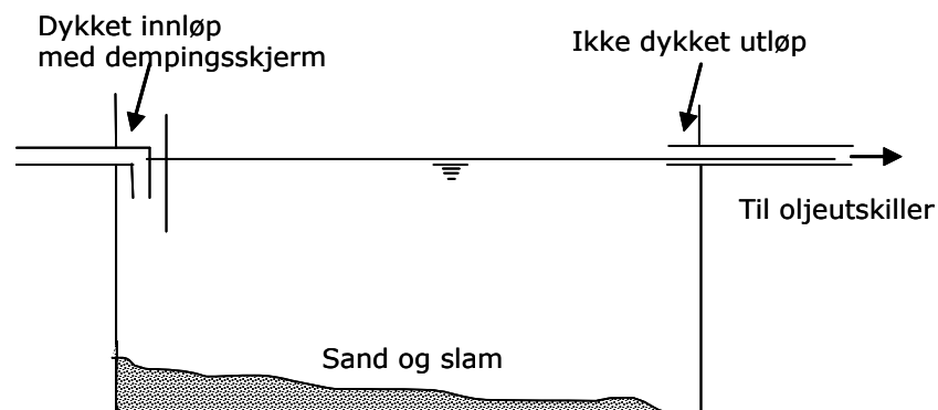
Figur 4.2 Skjematisk oppbygging av sandfanget
