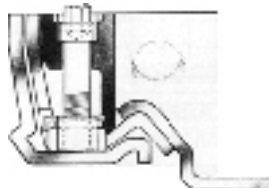
Låsebolt
